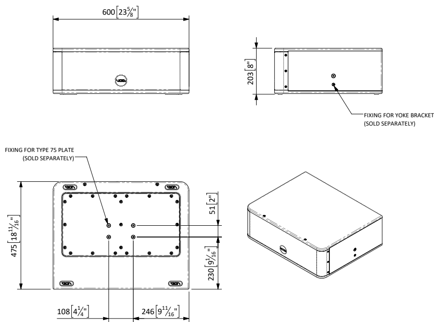
Figure B.10: Venu 208 V2 dimensions
